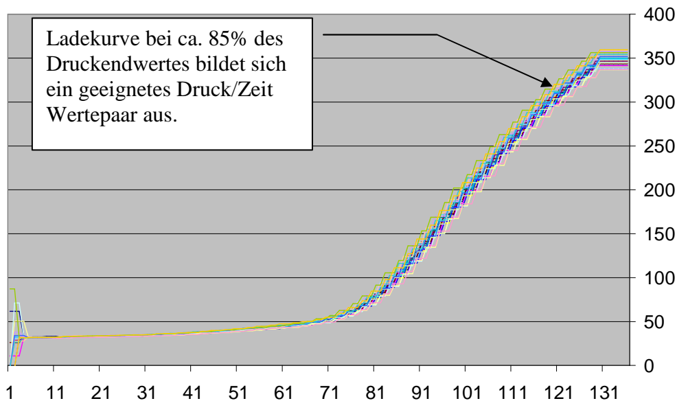
Bild Ladekurven (50 Messungen des gleichen Prüflings; x-Achse in 0,1s; y-Achse in mbar)
